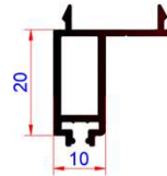
PROFILE # : AF-7307 DESCRIPTION : Sash Adapter WEIGHT : 0.738 KG/M
