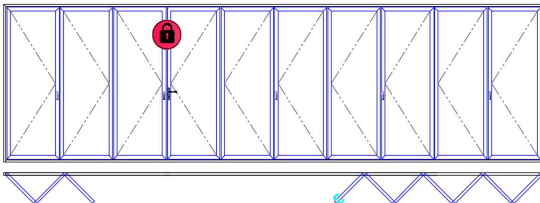
3+7 SASHS FOLDING DOOR
