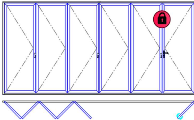
5+1 SASHES FOLDING DOOR
