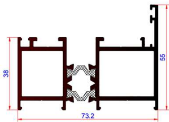
PROFILE # : AF-7301 DESCRIPTION : Frame WEIGHT : 1.75 KG/M
