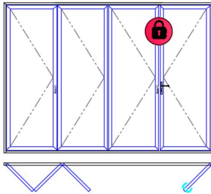
3+1 SASHS FOLDING DOOR
