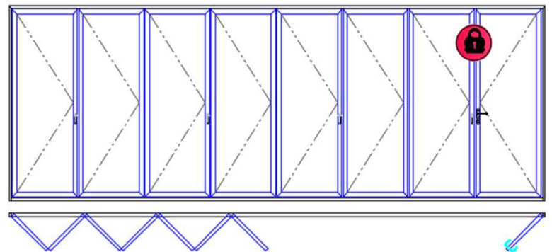
7+1 SASHES FOLDING DOOR
