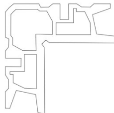
PROFILE # : AF-7314 DESCRIPTION : Sash Corner Cleat WEIGHT : 4.67 KG/M
