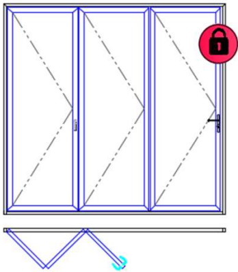
3 SASHS FOLDING DOOR
