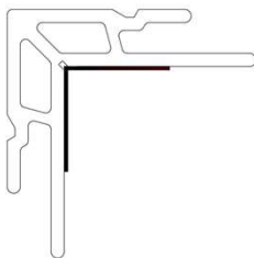
PROFILE # : AF-7315 DESCRIPTION : Frame Corner Cleat WEIGHT : 4.3 KG/M
