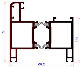
PROFILE # : AF-7302 DESCRIPTION : Horizontal Sash WEIGHT : 2.167 KG/M
