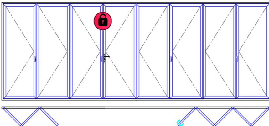
3+5 SASHS FOLDING DOOR
